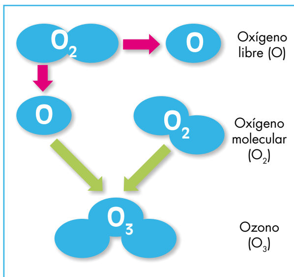
Representación gráfica de las moléculas de oxígeno.
