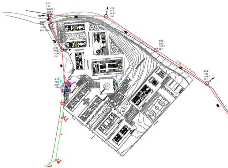
Figura 7: Parte de la red de medio voltaje proyectada
