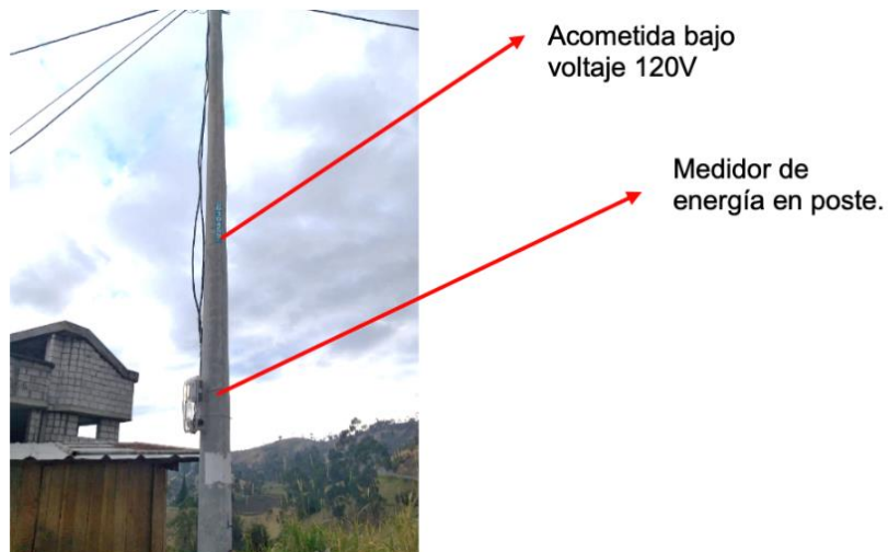
Figura 5: Acometida área de bajo voltaje
